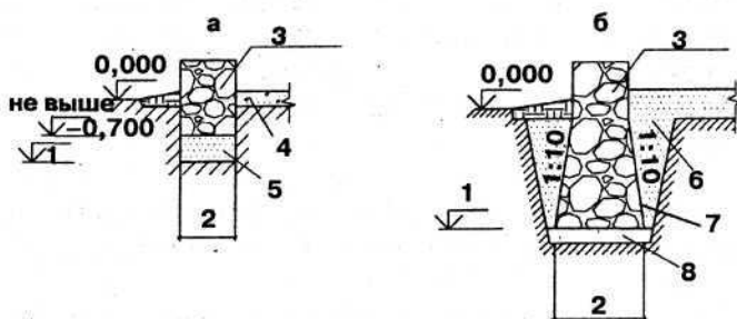
Рис. 5. Кладка бутобетонных фундаментов (не менее 35 см при ленточном фундаменте и не менее 40 см при столбчатом): а — в непучинистых грунтах; б — в пучинистых грунтах; 1 — расчетный уровень заложения фундамента; 2 — расчетная ширина фундамента; 3 — бутобетонный фундамент; 4 — подсыпка из грунта; 5 — подушка из крупнозернистого песка не менее 10 см; 6 — обратная засыпка грунтом; 7 — обмазка горячим битумом; 8 — опорная подушка из уплотненного грунта не менее 10 см
