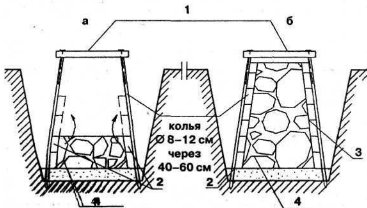
Рис. 13. Схема устройства опалубки для бутобетонного фундамента при бетонировании:
