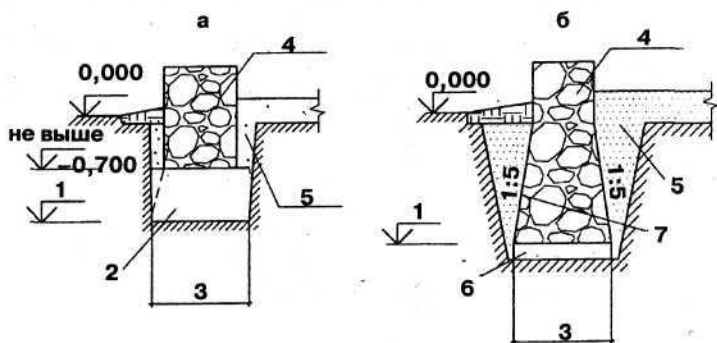
Рис. 4. Возведение бутовых фундаментов (не менее 50 см при ленточном фундаменте и не менее 60 см при столбчатом): а — в непучинистых грунтах; б — в пучинистых грунтах; 1 — расчетный уровень заложения фундамента; 2 — подушка из крупнозернистого песка не менее 10 см; 3 — расчетная ширина фундамента; 4 — бутовый фундамент; 5 — обратная засыпка грунтом; 6 — опорная подушка из уплотненного грунта не менее 10 см; 7 — штукатурка цементным раствором и обмазка горячим битумом
